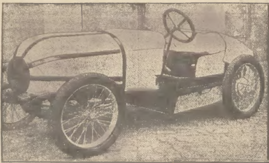
(—) Inżynier niemiecki Graichen skonstruował samochód gazowo-turbinowy. Turbina ta pracuje najtańszymi środkami opalowymi i może być również użyta do napędu samolotów i okrętów.
