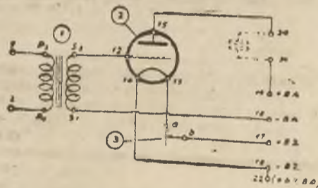
Rys. 2. Schemat teoretyczny.
