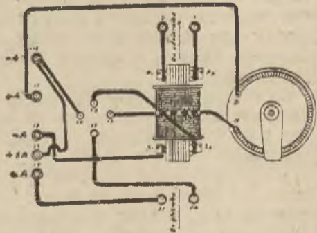
Rys. 1. Schemat montażowy.
