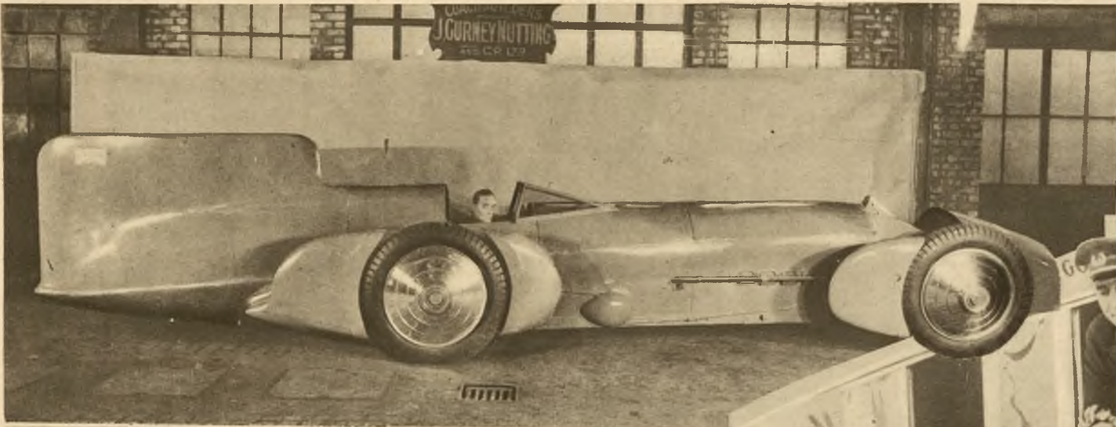
Angielski kapitan Campbell w swoim „Blue-birdzie” o 1.450 H. P., którym postanowił pobić światowy rekord szybkości jazdy automobilem.
