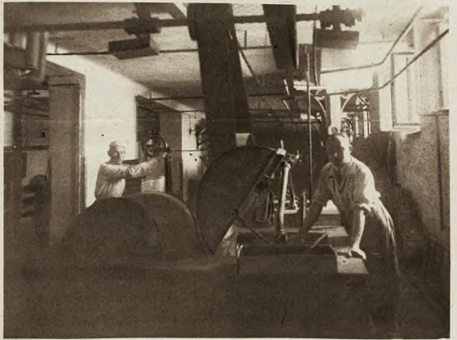
Hala maszyn (Conche i kompressor)
