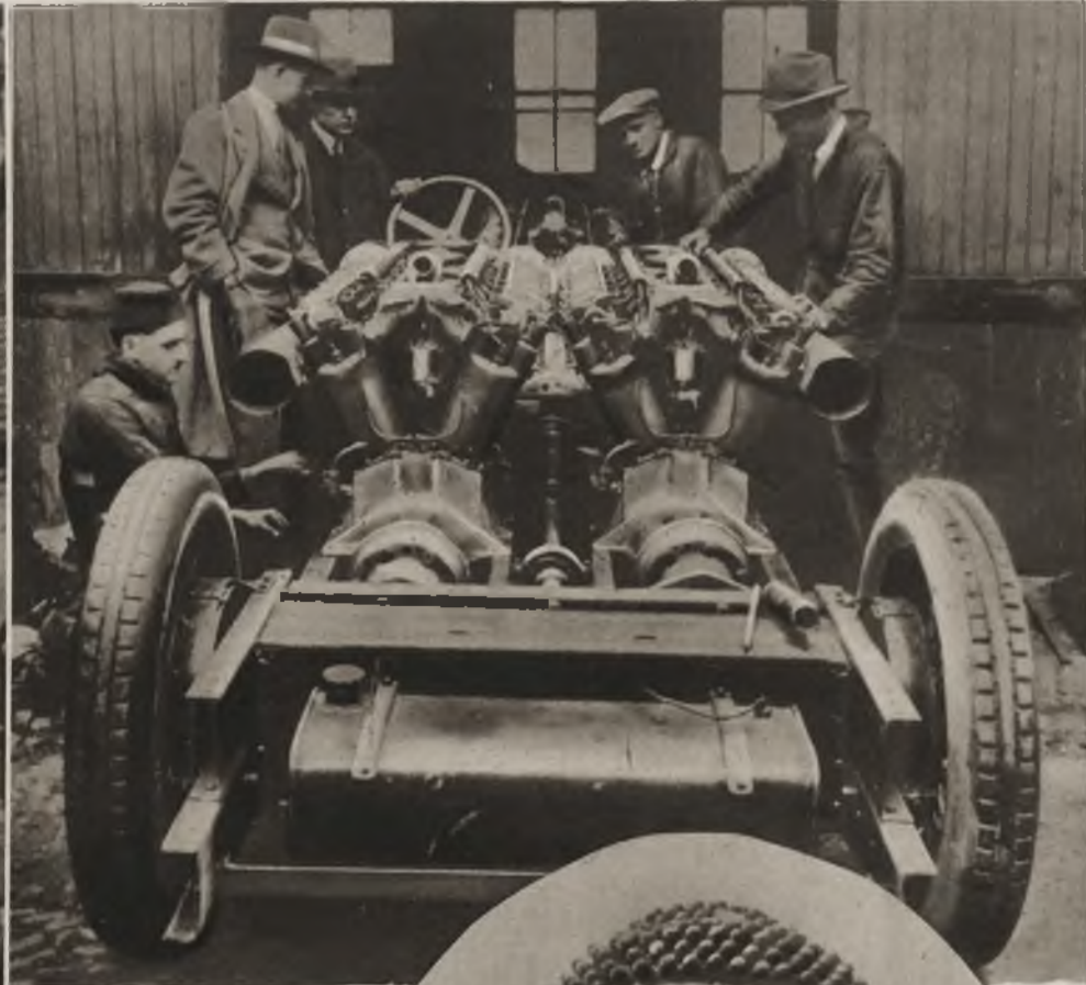
I. M. White z Filadelfji, zbudował auto, na którym zamierza pobić rekord Segrave'a. Wóz zw. Triplex, posiada 3 motory, każdy po 12 cylindrów. Z tych 2 są umieszczone z tyłu, 1 z przodu. Maszyna waży 4 tony.
