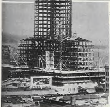
Budowa nowego olbrzymiego magistratu w Los Angeles. Na zdjęciu widoczne kompletne rusztowanie stalowe drapacza chmur, które potem oblewa się betonem.
