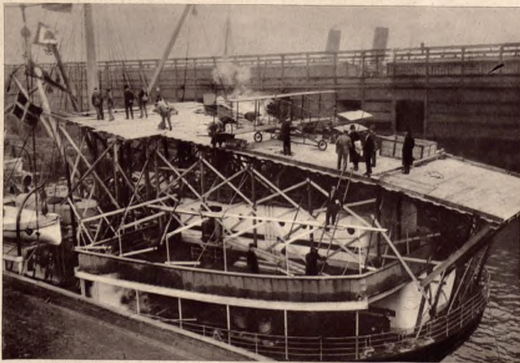
Powyższe zdjęcia wykazują postęp techniki jaki zastosowano przy starcie samolotów pocztowych z pokładu jadącego okrętu. Na lewo start w r. 1910 wymaga olbrzymiego rusztowania i przygotowań w przeciwieństwie do okrętu Bremen który wysłał samolot przy pomocy urządzenia katapultowego.
