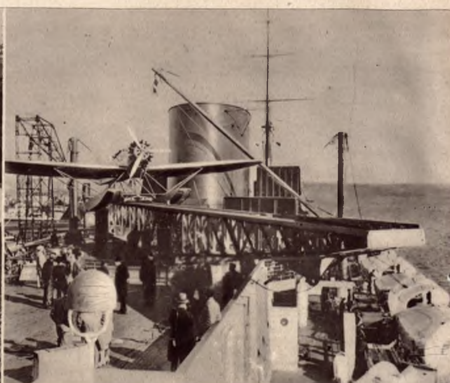
Powyższe zdjęcia wykazują postęp techniki jaki zastosowano przy starcie samolotów pocztowych z pokładu jadącego okrętu. Na lewo start w r. 1910 wymaga olbrzymiego rusztowania i przygotowań w przeciwieństwie do okrętu Bremen który wysłał samolot przy pomocy urządzenia katapultowego.
