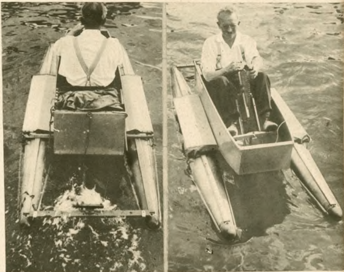
Najnowszy typ sani wodnych lansują obecnie w Niemczech. Wprawia się je w ruch za pomocą koła zębatego poruszanego ręką, steruje przy pomocy nóg.
