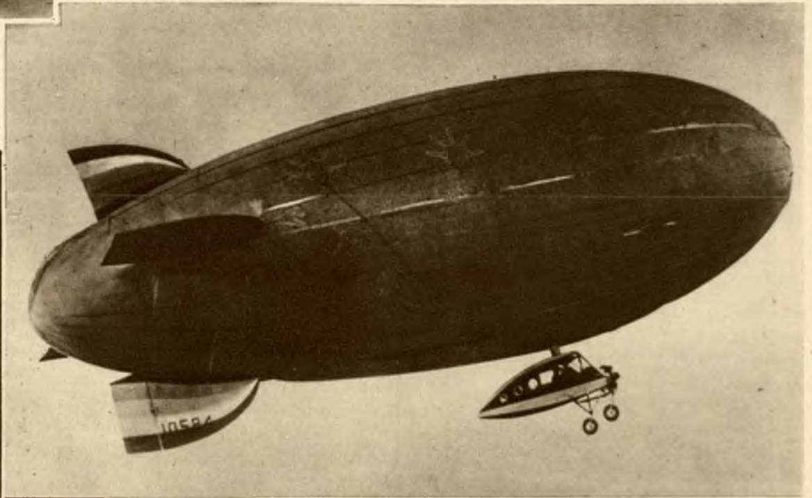
Jacht powietrzny zbudowany przez kap. Aton Heinen podczas swego pierwszego lotu w New Jersey (Stany Zjednoczone Ameryki).
