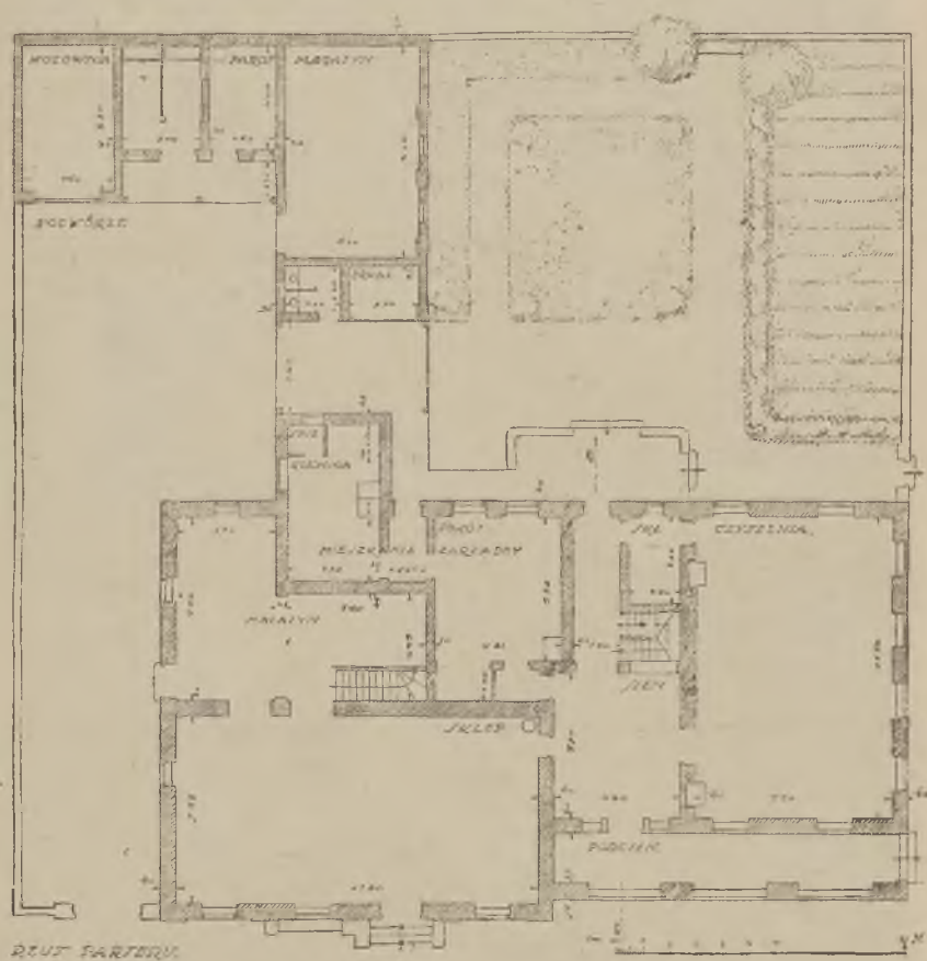
Ryc. 6. Inż. Józef Pokutyński. Dom ludowy (rzut parteru).
