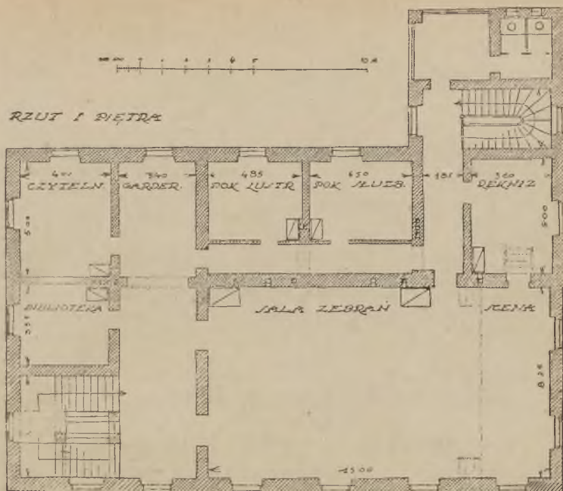
Ryc. 4. Inż. Zygmunt Harland. Dom ludowy większy (rzut I. piętra).
