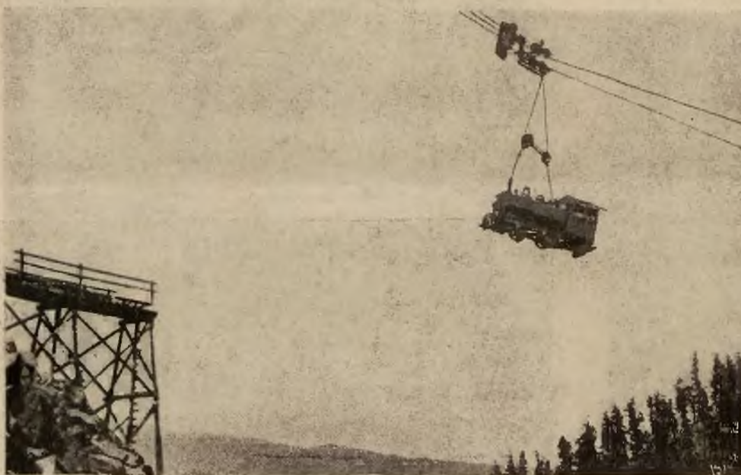
Rząd Stanów Zjednoczonych buduje obecnie wielką grębłę koło Rim Rock (Washington). Lokomotywy i materiał budowlany przewozi się kolejką linową nad głęboką przepaścią.
