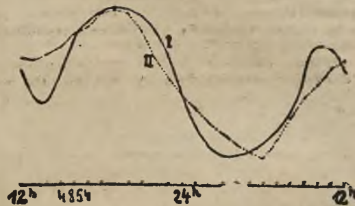
Ryc. II. Linja oznaczona przez I, przedstawia przeciętną częstość trzęsień ziemi w ciągu dnia. Linja II, przedstawia przeciętne odchylenia szybkości ziemi od normy. Zgodność obu linii wykazuje, że naogół ilekroć ruch ziemi staje się nieregularny, tylekroć występują trzęsienia ziemi.
