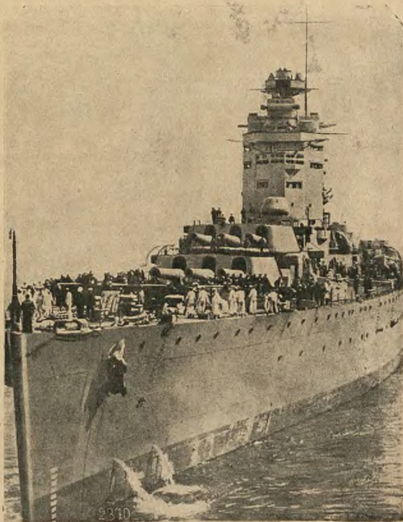
Najpotężniejszy pancernik świata, angielski okręt wojenny „Rodney“ niedawno ukończony i spuszczonej na wodę. Uzbrojony jest w trzy wieże, każda wieża posiada trzy armaty kalibru 406.
