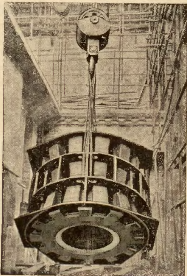
Część wielkiego turbogeneratorsa wykonana przez fabrykę niemiecką dla Japonii. Ciężar tego turbo-generatora wynosi 110 tonn.
