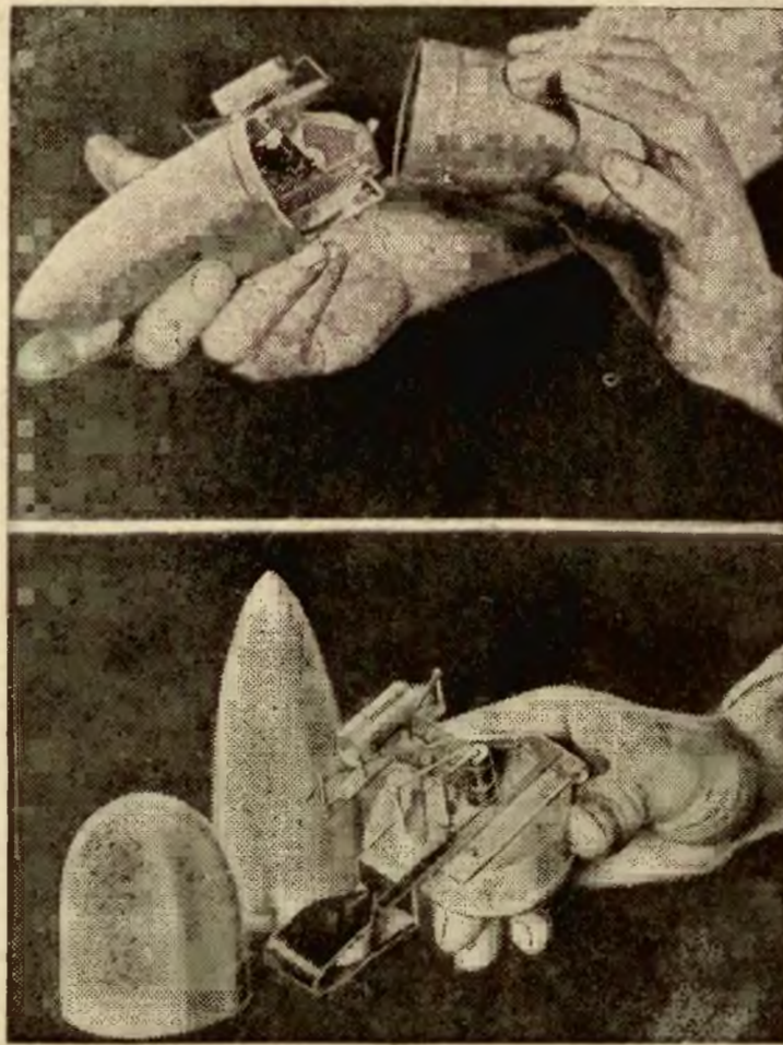
Harvard Blue Hill — Obserwatorium skonstruowało przyrząd nazwany meteorografem. Wewnątrz niewielkiej kapsli znajduje się termometr, barometr, i hydrometr. Aparat ten waży zaledwie trzy funty. Gdy samolot uniesie go w powietrze, przenosi on za pomocą fal krótkich co pół minuty zmiany temperatury, wilgoci i ciśnienia powietrza. Dany ten automatycznie notuje w obserwatorium chronograf.
