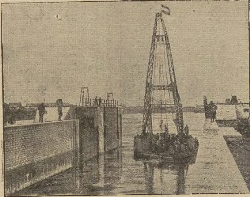
(dy) W tych dniach ukończono budowę pierwszej śluzy (nasza rycina) na jeziorze Znider. Służę tę zbudowano w celu osuszenia jeziora.
