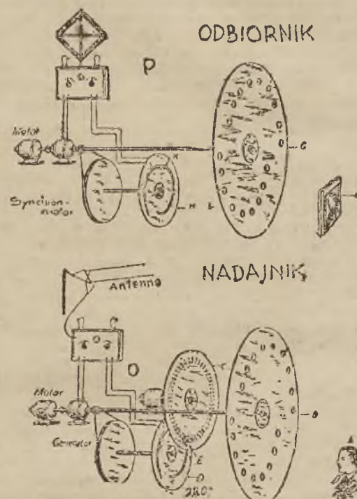
Rys. III. Schemat telewizora Bairda. A — nadawany przedmiot, B — tarcza wyposażona w spiralnie ku środkowi zbiegające się otwory zaopatrzone w soczewki, C — druga tarcza z otworami, szybko wirująca, D — tarcza wyposażona w spiralną szczelinę, E — przyrząd przenoszący „przecedzony” przez trzy tarcze B, C, D, promień na komercie fotoelektryczną, G — radjonadajnik, F — obraz na matówce, I, J, K tarcze wirujące, L — przyrząd z którego lampa neonowa wysyła światło różnej siły, P — radjoodbiernik.
