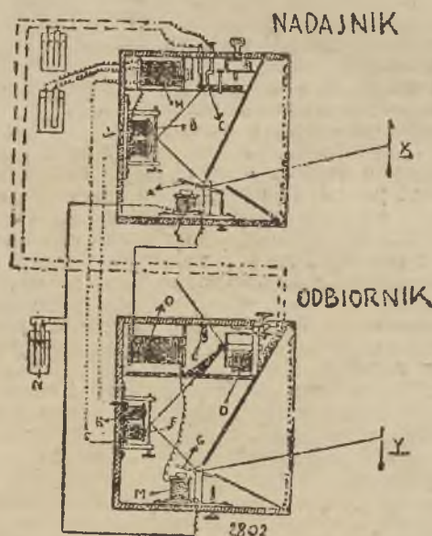
Rys. II. Schemat telewizora Szczepanika, X — przedmiot „nadawany”, A — pierwsze drgające zwierciadło, B — drugie drgające zwierciadło, C — płytkę selenu, D — elektromagnes, E — lampa elektryczna, do której dochodzi prąd przez płytkę selenu C F i G zwierciadła drgające synchronicznie z zwierciadłami A i B, Y — obraz na ekranie odbiornika.
