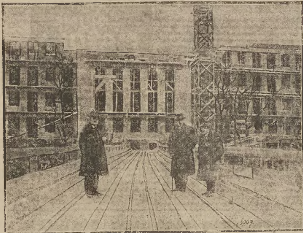
(d.) Budowa olbrzymiego gmachu Sanatorium Kasy Chorych m. Lwowa przy ul. Kurkowej. Rozpiętość frontu gmachu wynosi 87 metrów. Widok budowy z pomostu wieży drewnianej z wyciągami mechanicznymi. (Fotogr. red. Daniluk.)
