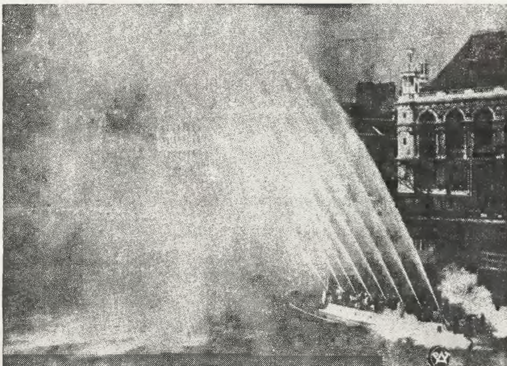
Angielski statek do gaszenia pożaru podczas próbnej akcji na Tamizie koło mostu Blackfriars.
