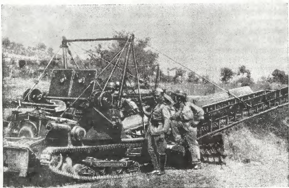
Na odbywających się we Włoszech manewrach wypróbowano nowy tank, który ma na sobie coś w rodzaju mostu, dzięki czemu przekraczać może rowy szerokie ponad 5 m.
