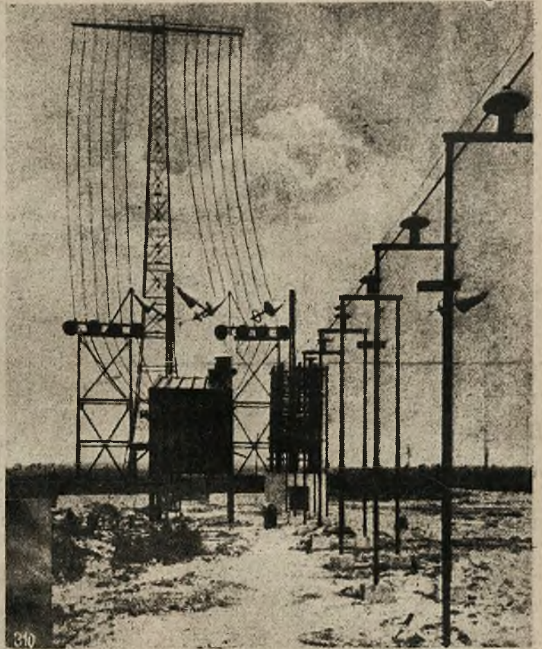
310 Amerykańska stacja nadawcza i odbiorcza niedawno zaprowadzonej komunikacji telefonicznej bez drutu między Ameryką i Anglią.
