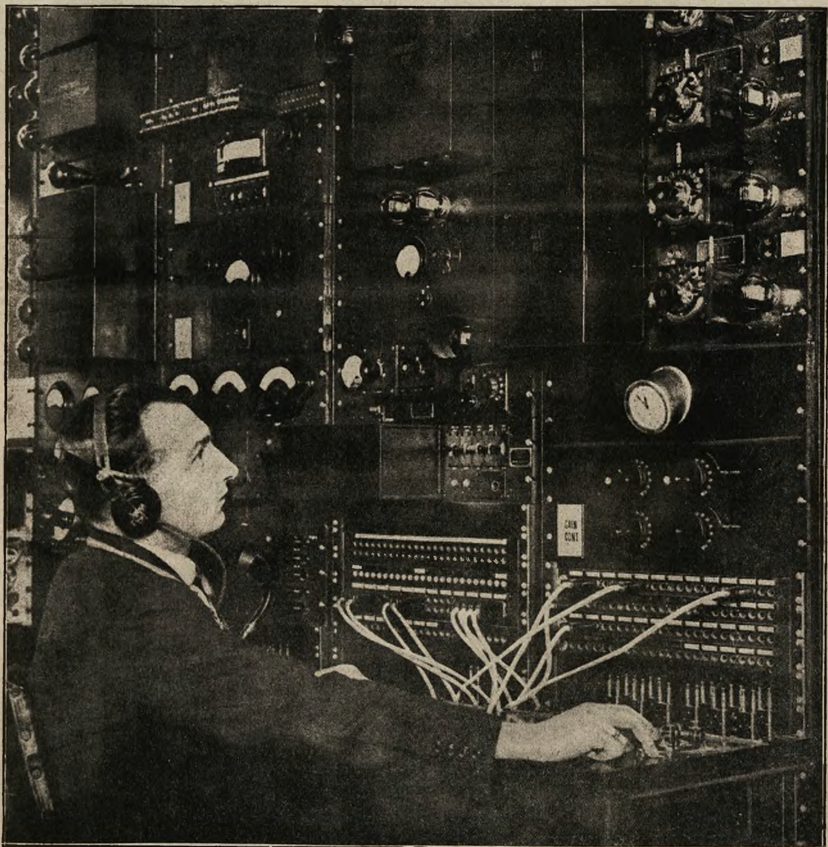
Centrala telefoniczna w Londynie dla rozmów przy pomocy telefonu bez drutu między Londynem a N. Jorkiem. Minuta rozmowy kosztuje 250 złp.
