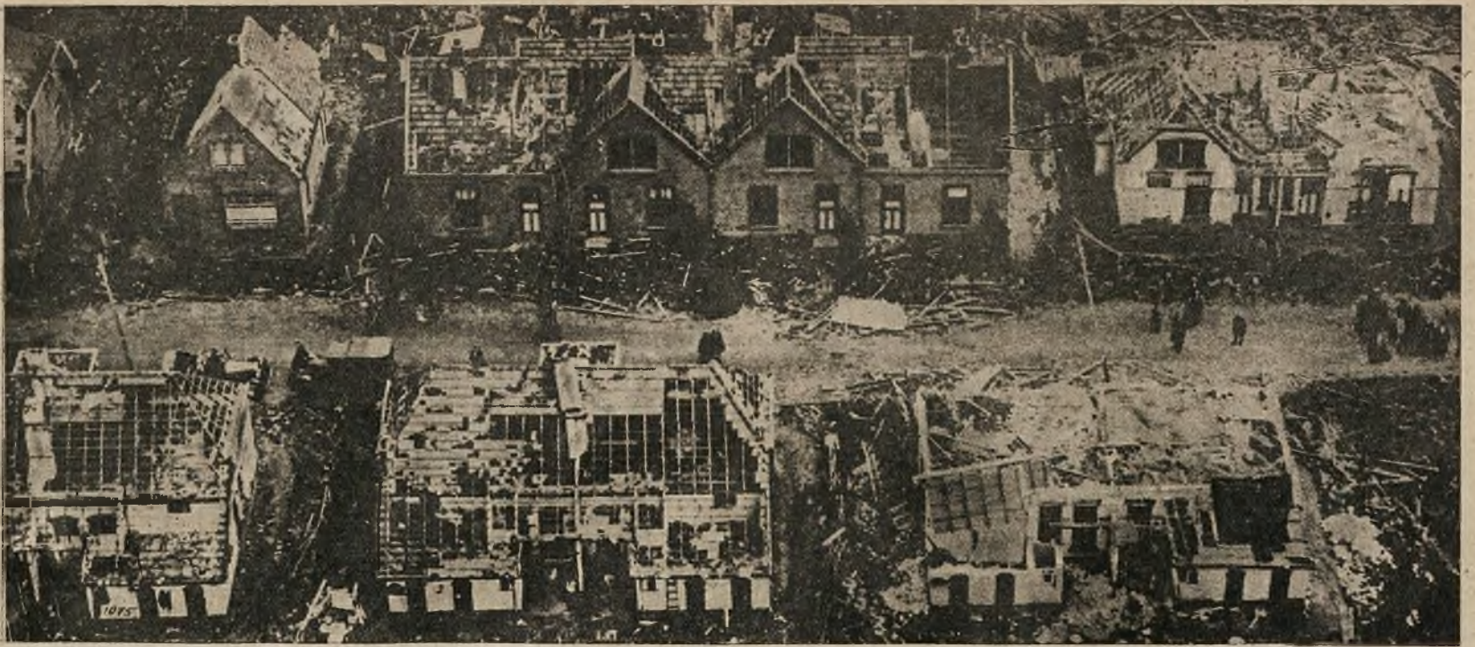
Olbrzymi cyklon zniszczył niedawno szereg miast w prowincji Golderland w Holandji. Rycina przedstawia zerwane dachy domów w mieście Neede.
