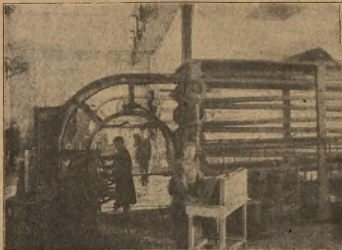
Maszyna „Ideal“ otrzymuje surowe pałyczki a wydaje gotowe zapalki.
