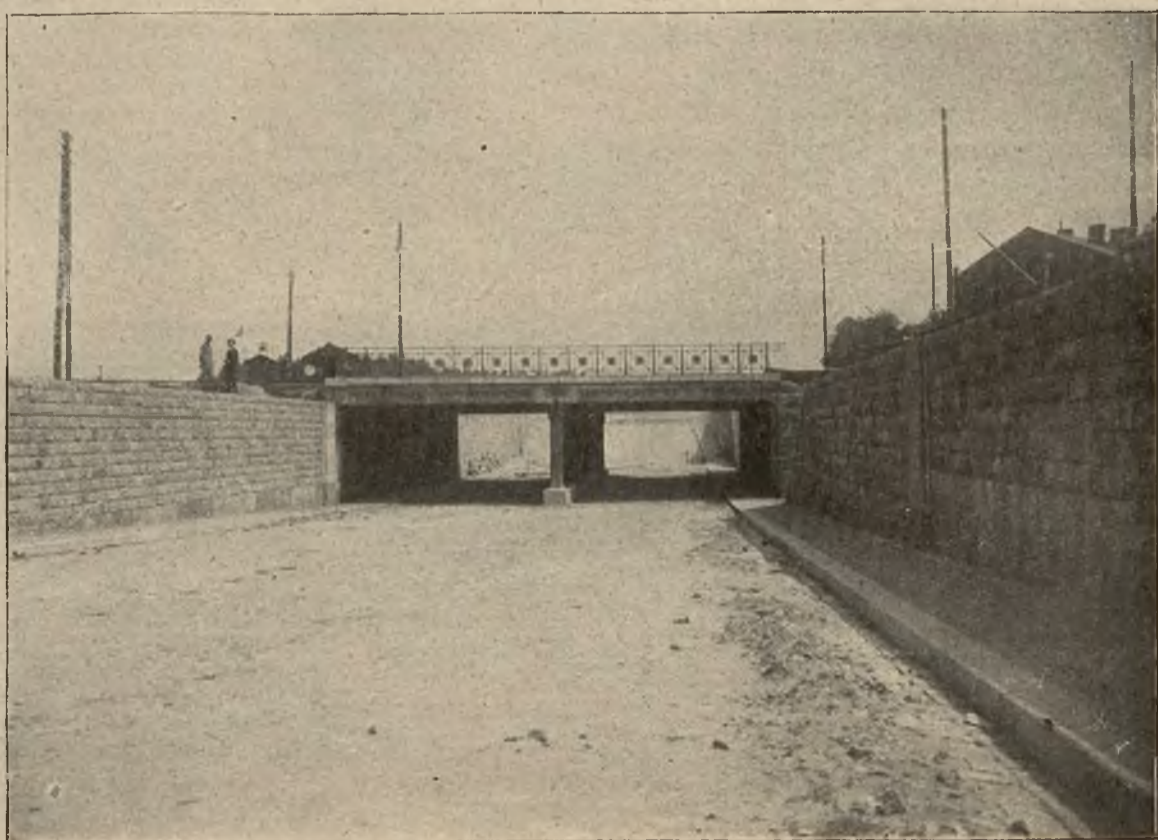
Nowy dworzec towarowy w Krakowie: Podkop na Krowodrzę i dojazd do przyszłych magazynów.
