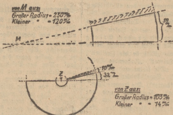
So wird das Blech für den Trichter vorgezeichnet
