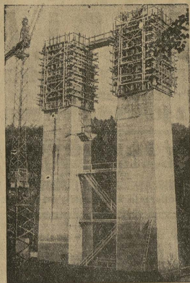
Z olbrzymim nakładem kosztów przystąpiła obecnie Niemcy do rozbudowy sieci swych autostrad. Zdjęcie przedstawia dwa potężne filary mostowe z betonu, na których spocznie wielki most na trasie autostrady nad doliną Mangfall w Bawarii. — Każdy z tych filarów ma 70 m. wysokości.
