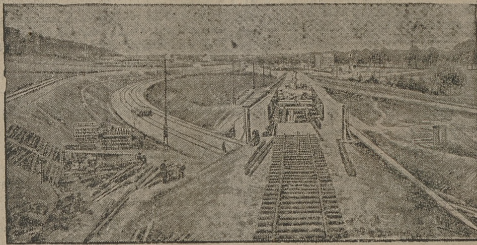
Ilustracja nasza przedstawia fragment budowy kolei G. Śląsk -- Gdynia.
