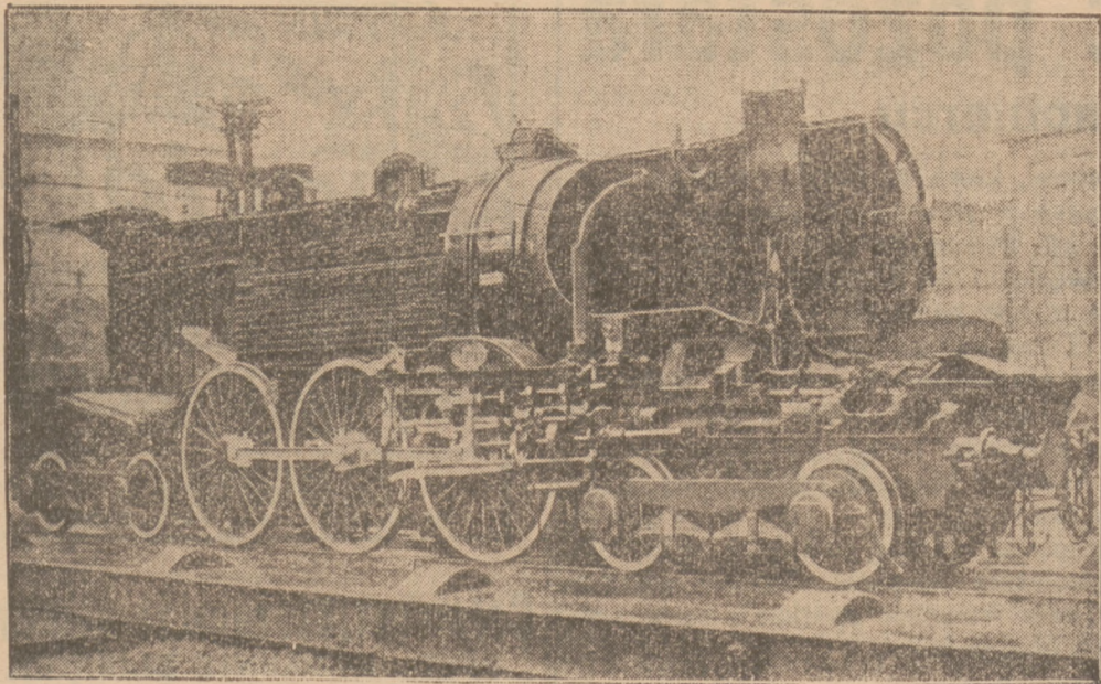
Jednym z oryginalniejszych eksponatów na wystawie światowej w Paryżu będzie przekrojona lokomotywa, której wewnątrz da laikowi możliwość zaznajomienia się z budową nowoczesnej lokomotywy.
