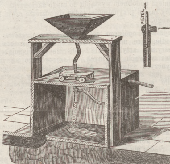
Przyrząd paropiaskowy.
