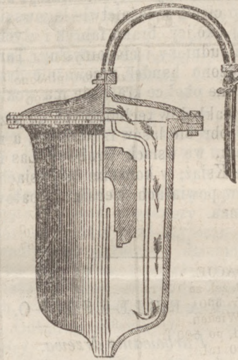
Fig. 58. Filtr wodociągowy.
