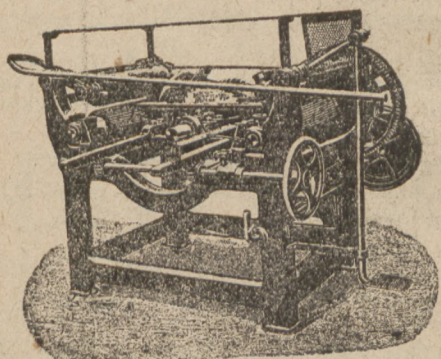
PODWÓJNA PIŁA TARCZOWA DKS
