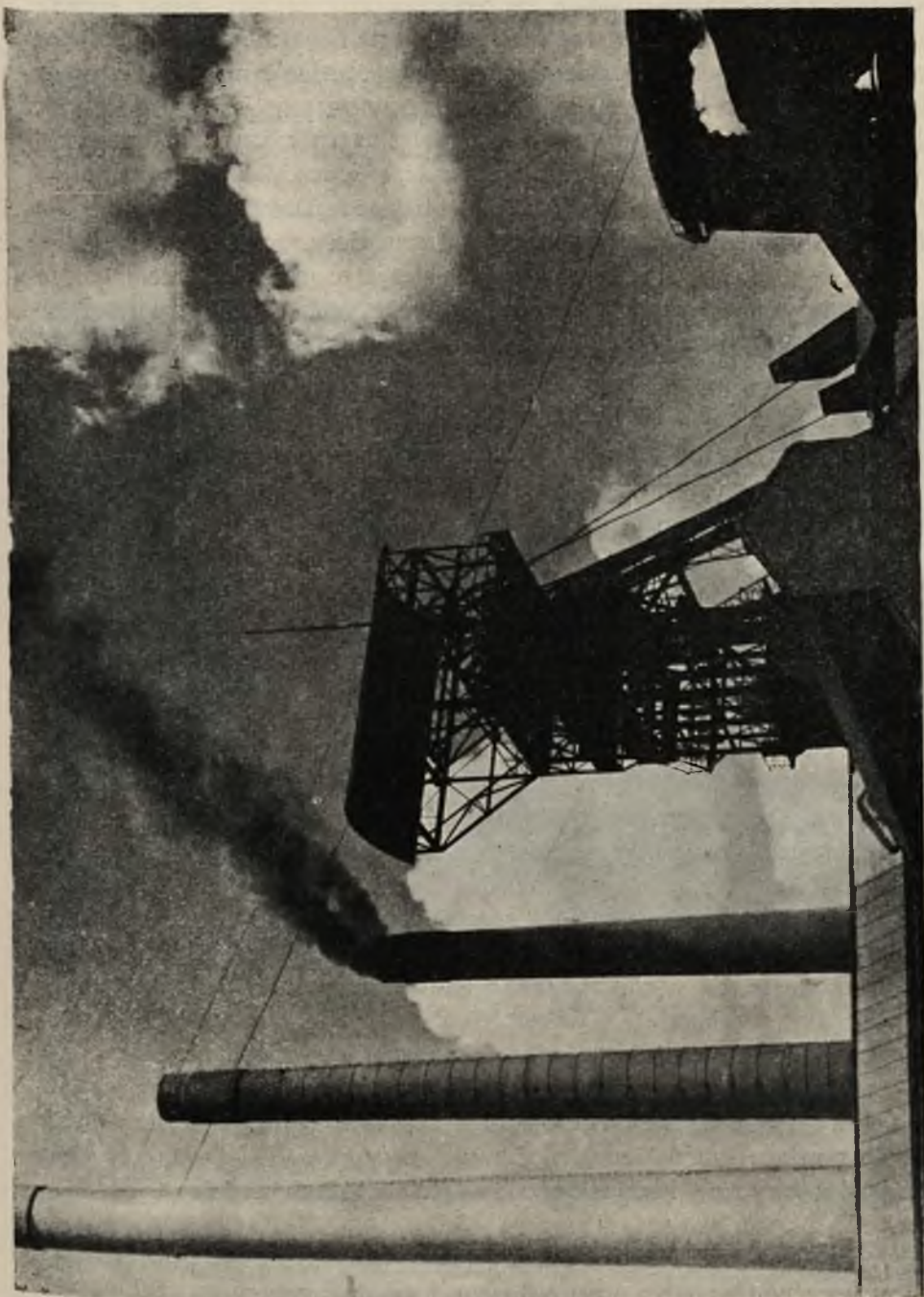
Wieża szysbu i kominy kopalni węgla w Zagłębiu Wałbrzyskim
