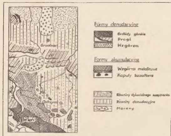
Mapka morfologiczna okolic Wlenia
