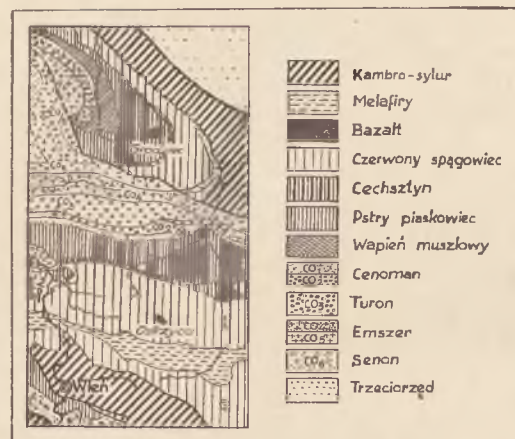
Mapka geologiczna okolic Wlenia
