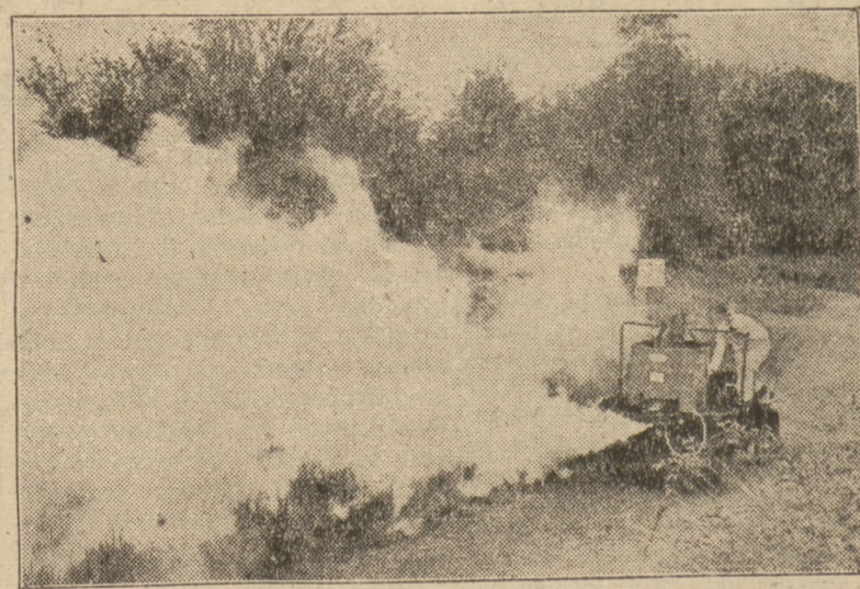
W Anglii wypróbowano nowy środek walki z moskitami — sztuczną mgłę owadobójczą, rozpylaną przy pomocy specjal- nego aparatu (SAP)
