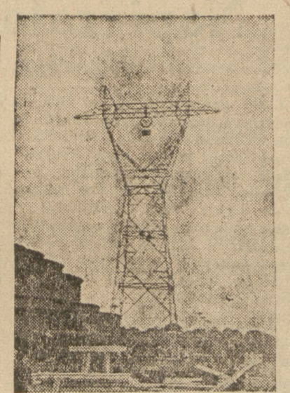
Zmontowany słup sieci wysokiego napięcia
