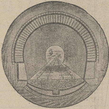
IZOLACJA TUNELU.
