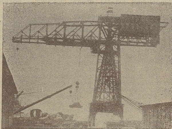
Nowozbudowany, największy w świecie dźwig okrętowy w Filadelfji.
