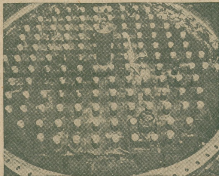
Uranium i ciężka woda w laboratorium Argonne blisko Chicago. Materiały które mają przejść proces radio-aktywności spuszczone są przez środek reaktora do ciężkiej wody.
