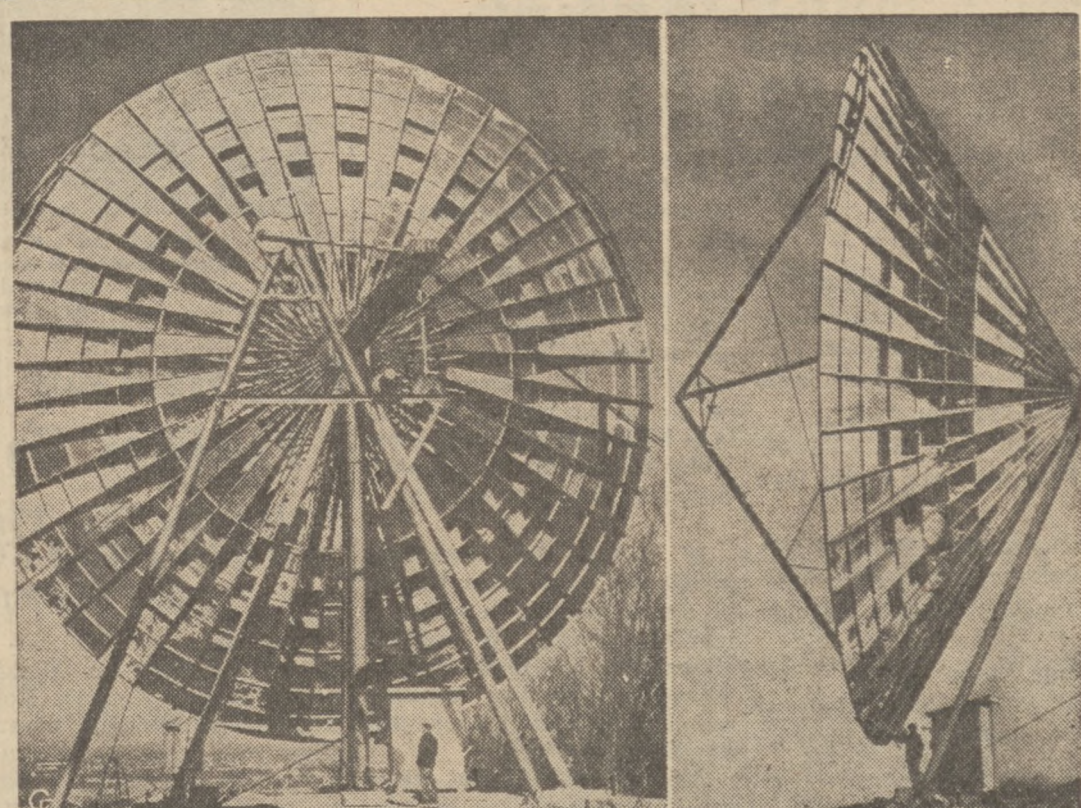
NAJWIEKSZA ANTENA ŚWIATA — Na wzgórzu w pobliżu Holmdel, N. J. wybudowano specjalną antenę o wysokości 60 stóp, która może odbierać sygnały telefoniczne i telewizyjne nadawane z odległości 20 mil. Instytut Techniczny Massachusetts i laboratoria kompanii Bell Telephone podają do wiadomości, że został już rozwiązany problem transmisji telewizyjnych na wielkie odległości przy zastosowaniu specjalnie wysokiej częstotliwości fal.
