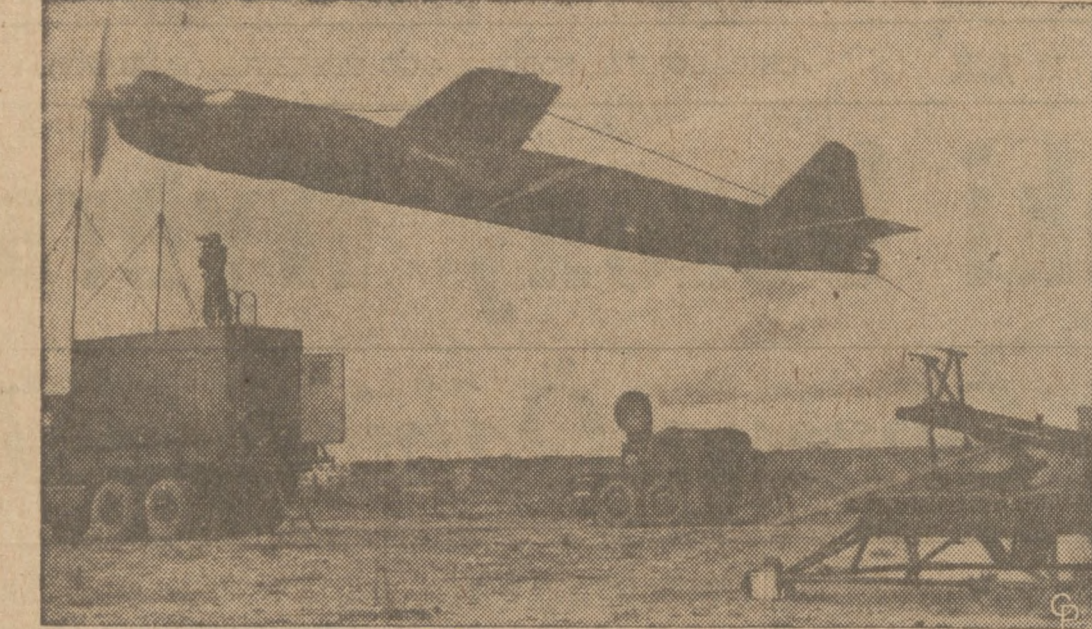
NIEZWYKŁY SAMOŁOT. Powyżej widzimy automatyczny samolot amerykański używany do fotografowania terenów nieprzyjacielskich. Samolot kierowany jest dystansowo przy pomocy specjalnego aparatu. Osobliwością samolotu jest to, iż dokonuje on fotografii w nocy.
