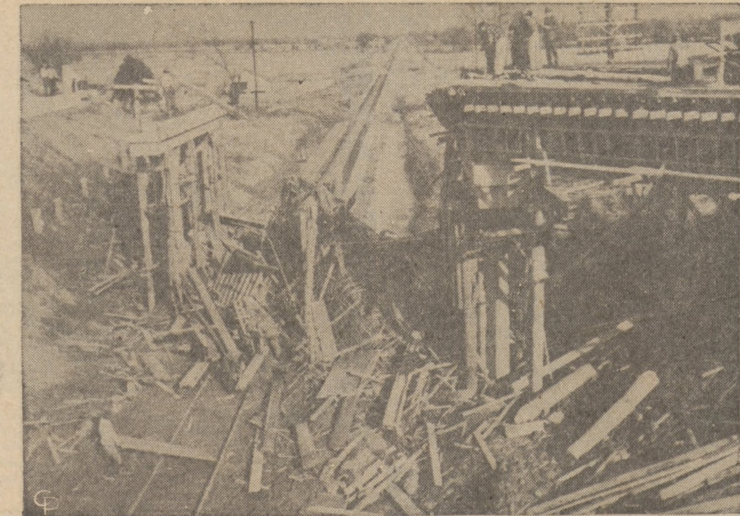
COS TU ZAWINIŁO. — W czasie budowy mostu ponad przejazdem kolejowym niedaleko Memphis, Tenn., w chwili gdy poczęto wlewać cement, załamała się gotowa już konstrukcja żelazna i wszystko runęło w dół, zabierając z sobą również i 7 robotników. Jeden z nich jest tylko ciężko ranny. Robota kosztowała już pół miliona dolarów.
