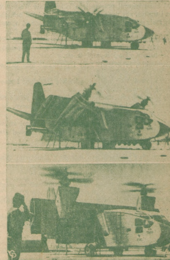
OCZEKUJE PRÓB. Nowy samolot doświadczalny typu X-18 oczekuje na lotnisku w Bazie Lotnictwa Edwards Base w Kalifornii na przeprowadzenie lotów próbnych. Samolot ten może startować pionowo, a po osiągnięciu pewnej wysokości, lecąc normalnie. Umożliwia to przestawianie odpowiednio skrzydeł wraz z wmontowaniem w nich silnikami.
