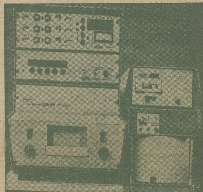
DO BADAŃ RADIOAKTYWNOŚCI W MLEKU. —Administracja od spraw żywności i lekarstw w Stanach Zjedn. przeprowadza obecnie w 11-tu miastach w kraju badania zawartości radioaktywnego skażenia w mleku, używając do tego instrumentów jak na zdjęciu. Aparat zdolny jest wykazać obecność już nawet 1 mikromikro-kura w litrze mleka lub wody. Defektory są produktami Laboratorium Sharp w La Jolla, Kalif.
