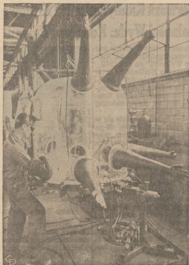
PRACA PRZY KAPSULE GEMINI — W zakładach McDonnell Aircraft w St. Louis wykańcza się konstrukcja kapsuły Gemini do lotu dwóch astronautów w Przestworza. Powyżej widać spawacza który spawa poszczególne części kapsuły Gemini, używając do swej pracy gumowych ręk. Spawanie części musi mieć miejsce w bez-powietrznej komorze.
