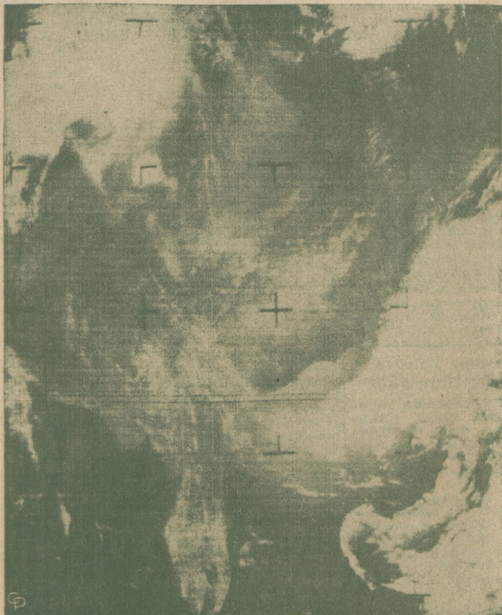
WSCHODNIA CZĘŚĆ STANÓW ZJEDNOCZONYCH. — Satelita do przekazywania pogody, Nimbus-2, obecnie wyrzucony w orbitę przesał zdjęcie wschodniej części Stanów Zjednoczonych. Na zdjęciu tym widzimy dokładnie Wielkie Jeziora (poniżej w środku), Chesapeake Bay (na prawo w środku), Florydę (niżej w środku) i Gulf of Mexico (u dołu z lewej). Nimbus-2, o wadze 912 funtów, został wyrzucony w orbitę z Vandenberg Bazy, California. Okrąża on ziemię z północy na południe i może fotografować wszystko na powierzchni ziemi w obrębie 200 milionów kwadratowych mil nawet w nocy. Spodziewane jest, że przy jego pomocy będzie można dokładniej przewidzieć zmiany pogody.
