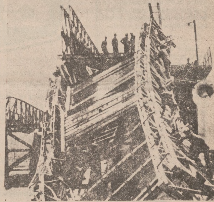
POŁUDNIOWY WIETNAM. — Inżynierowie południowo-wietnamscy studiują plan naprawy mostu w prowincji Binh Dinh, który podobnie jak wiele innych mostów w strefie sągoniskiej, został wysadzony w powietrze przez komunistów północno-wietnamskich.
