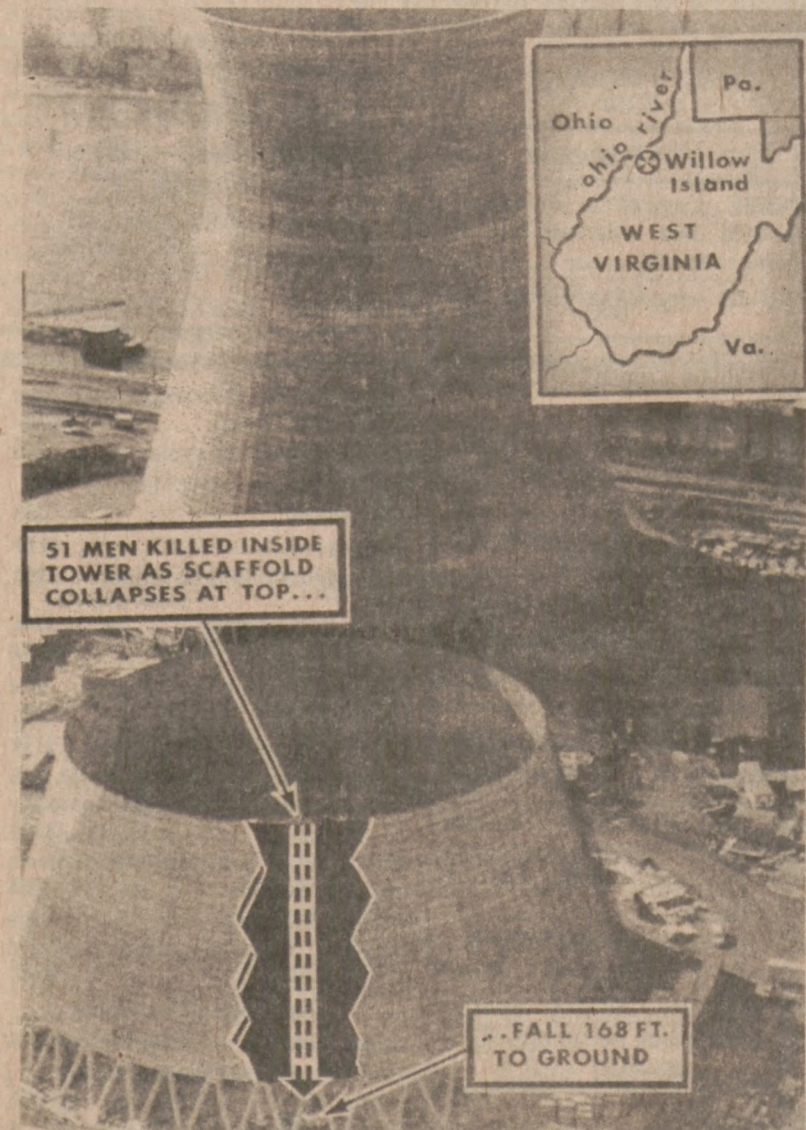
WILLOW ISLAND, W. VA. — Zdjęcie to przedstawia widok miejsca katastrofy zawalenia się rusztowania na wieży do chłodzenia wody. W katastrofie tej zginęło 51 osób. (UPI)
