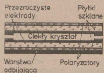
Konstrukcja segmentu wskaźnika ciekłokrystalicznego
