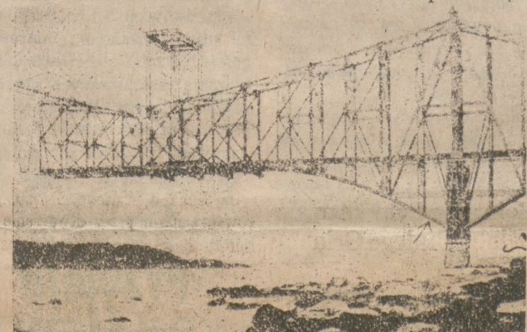
19. Pierwotna konstrukcja mostu w Quebec w dzień przed katastrofą. Strzałka wskazuje pręt, który był bezpośrednią przyczyną awarii
