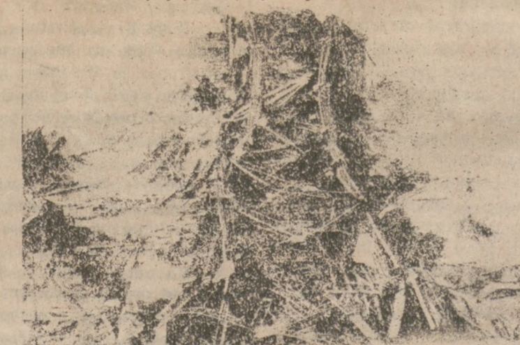
20. Widok konstrukcji mostu Quebec po katastrofie w dniu 29 sierpnia 1907
