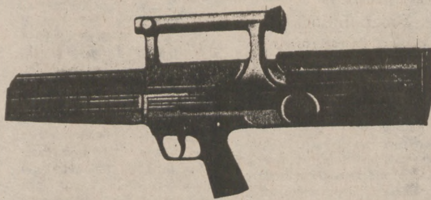
Automatyczny pistolet G-11 z magazynkiem na 50 bezłuskowych nabo, umieszczonym nad lufą. Celownik optyczny jest jednocześnie wygodną rączką.
