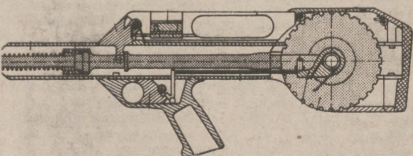
Współczesny australijski karabin-revolver z bębnowym jednorazowym magazynkiem na 30 bezłuskowych nabo, zakładanych do wnętrza kolby. Rewolwerowe rozwiązanie magazynku eliminuje problem samozapalony gdyż nie wprowadza się naboów do rozgrzanej komory naboowej, jak w rozwiązaniach pistoletowych.
